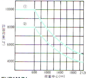
FVD135Z4
