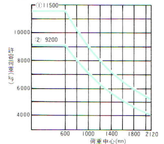
FVD115Z4
