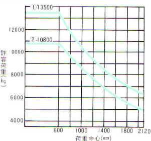
FVD135Z4
