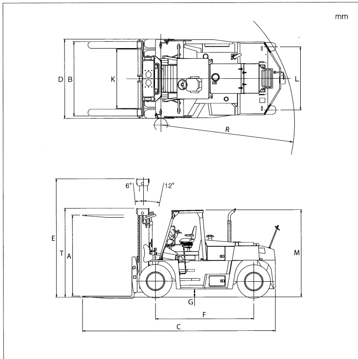
外形寸法図
