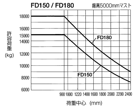
荷重表
