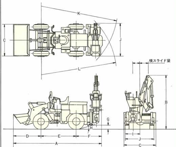
トラクタショベル STD10/STD25/45
