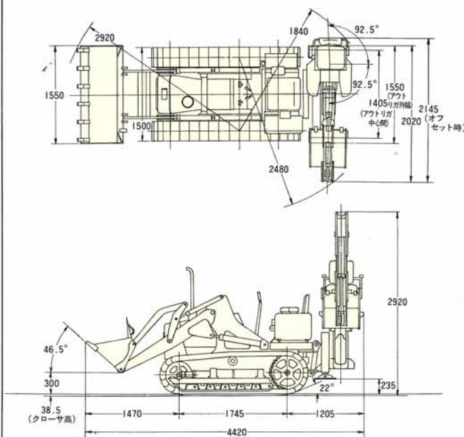
クローラショベル SCD10
