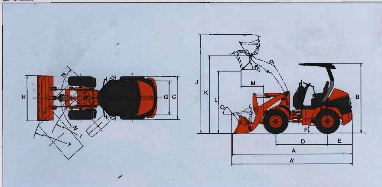
■ 寸法図
