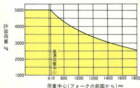
荷重表
