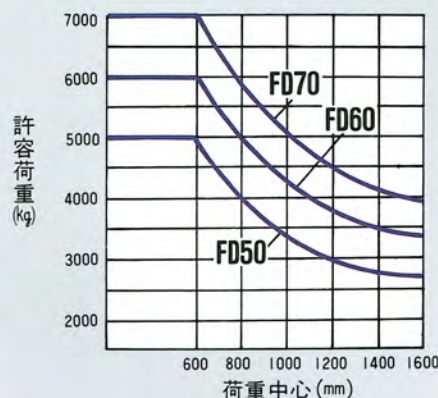
■荷重表
