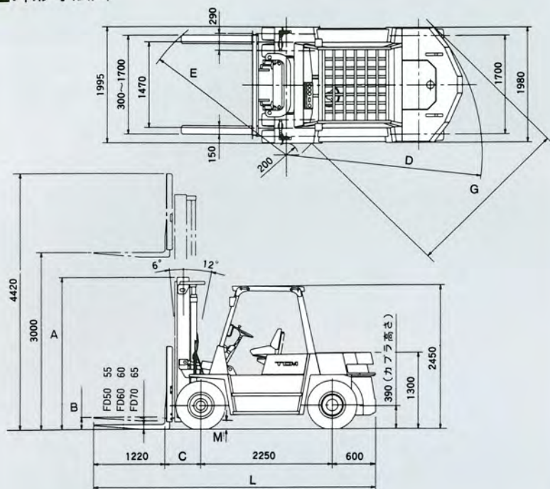
■外形寸法図
