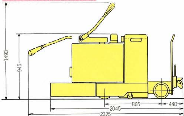
無人けん引車 (ATB20)
