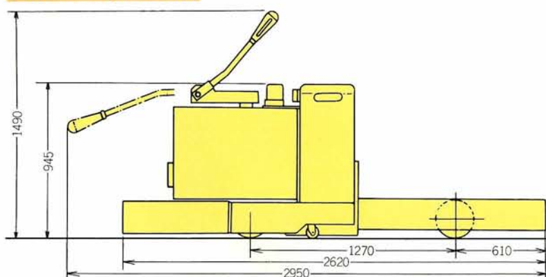
無人台車 (AWB10)
