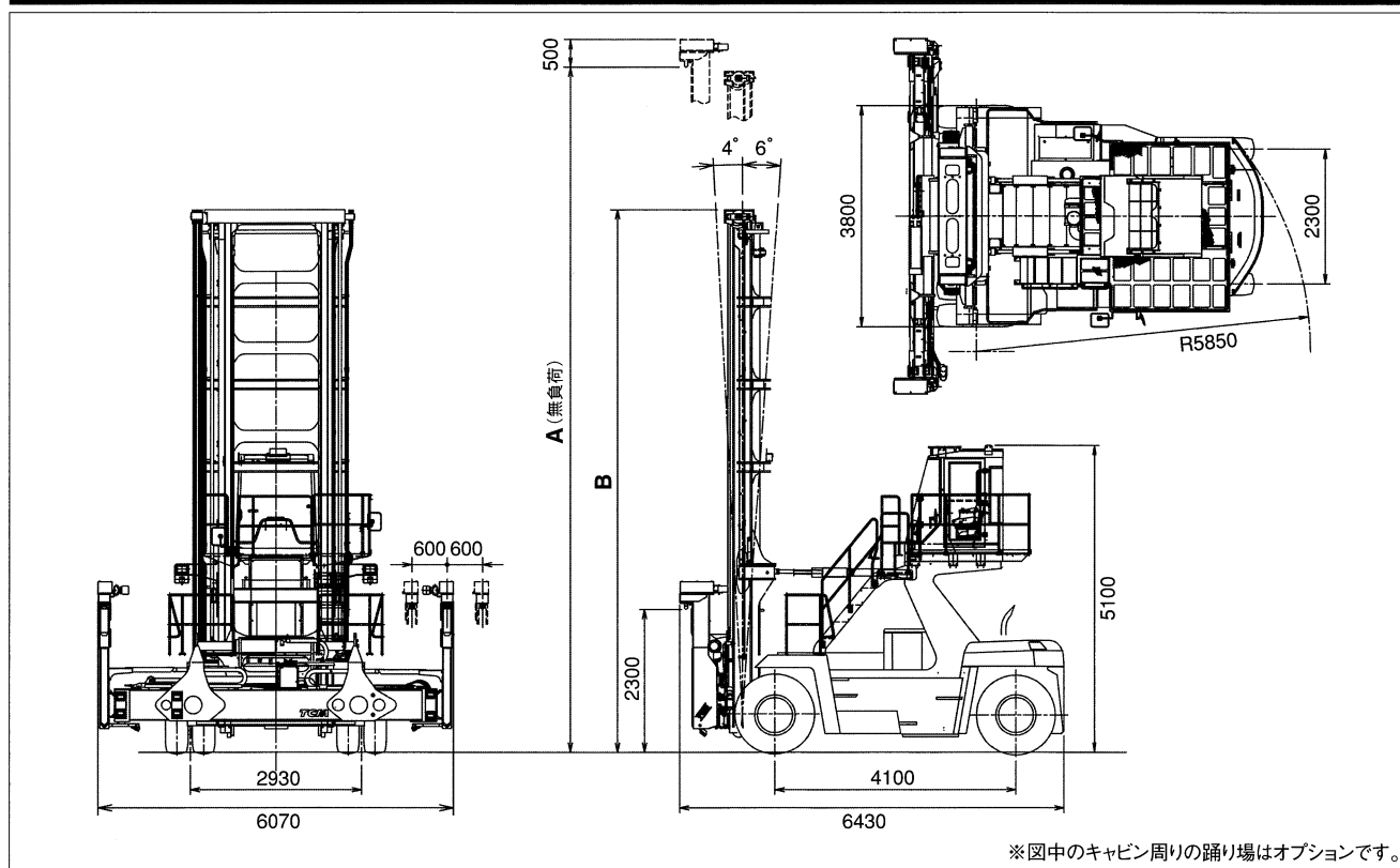
外形寸法図
