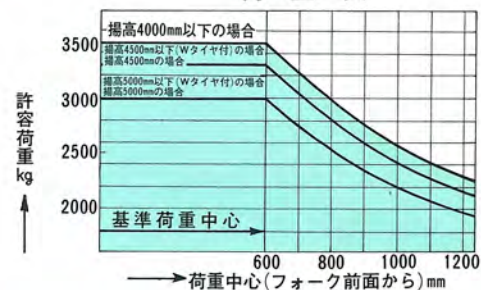
荷重表
