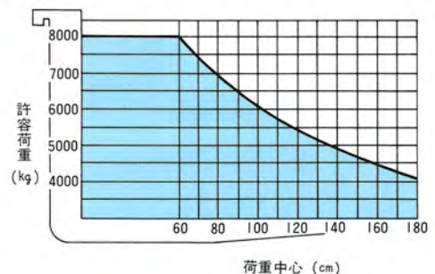
荷重表
