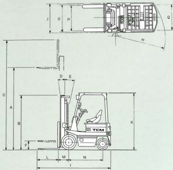
■外形寸法図
