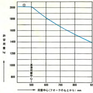
荷重表
