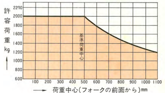
荷重表
