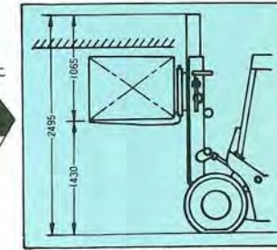
標準マスト(M300)
