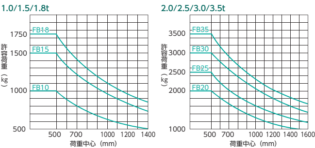
■ 荷重表
