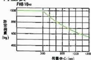
荷重表
