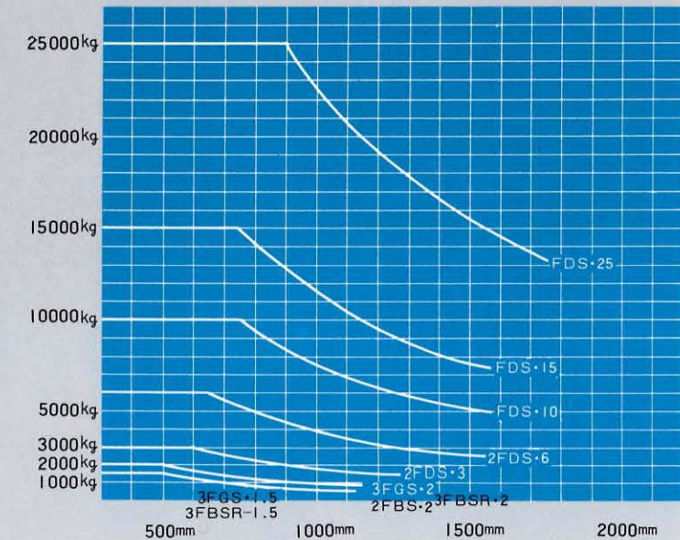
荷重曲線
