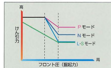
■新油圧回路によるスムーズな複合動作が可能
