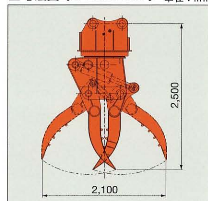
■寸法図 (S-FG65-RT)
