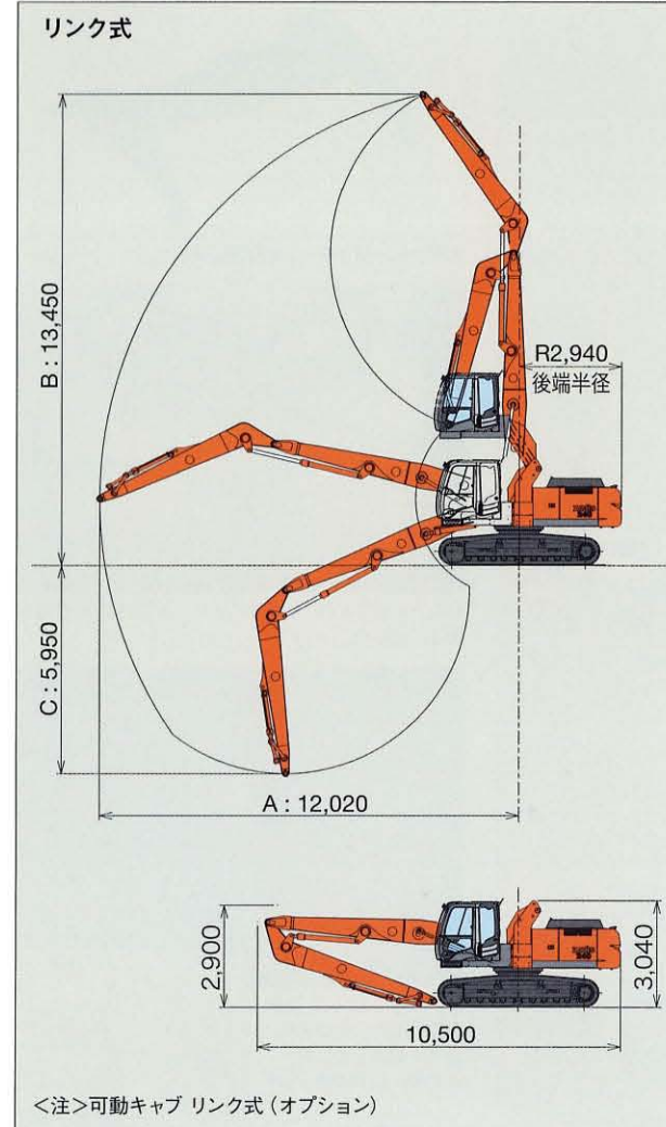
■作業範囲図 (ZX240LC-3)
