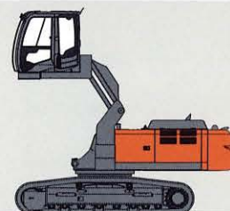
■可動キャブ リンク式
