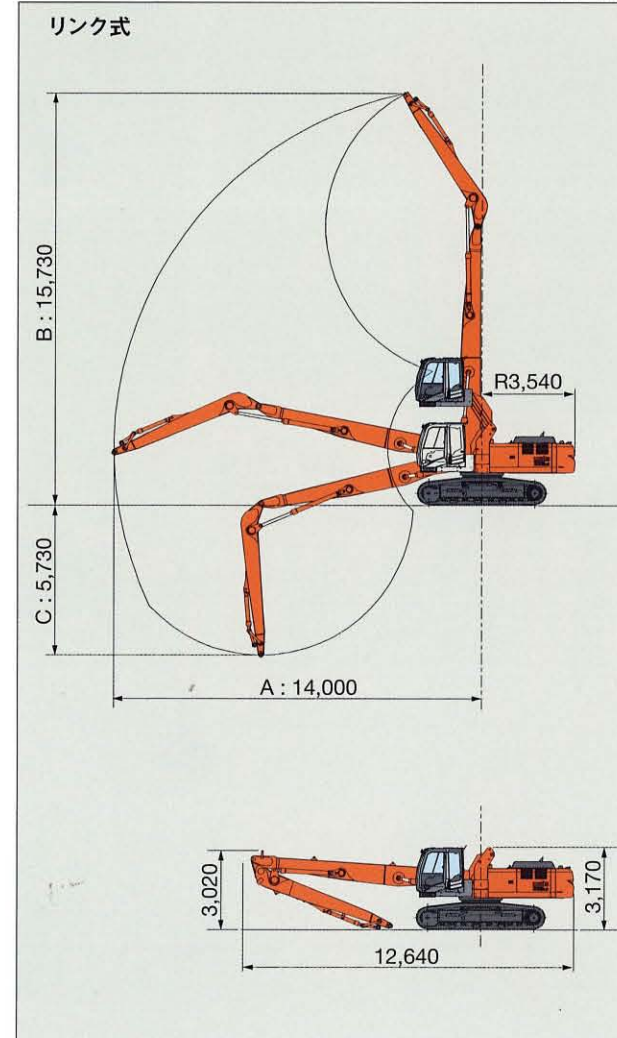
■作業範囲図 (ZX330LC-3)
