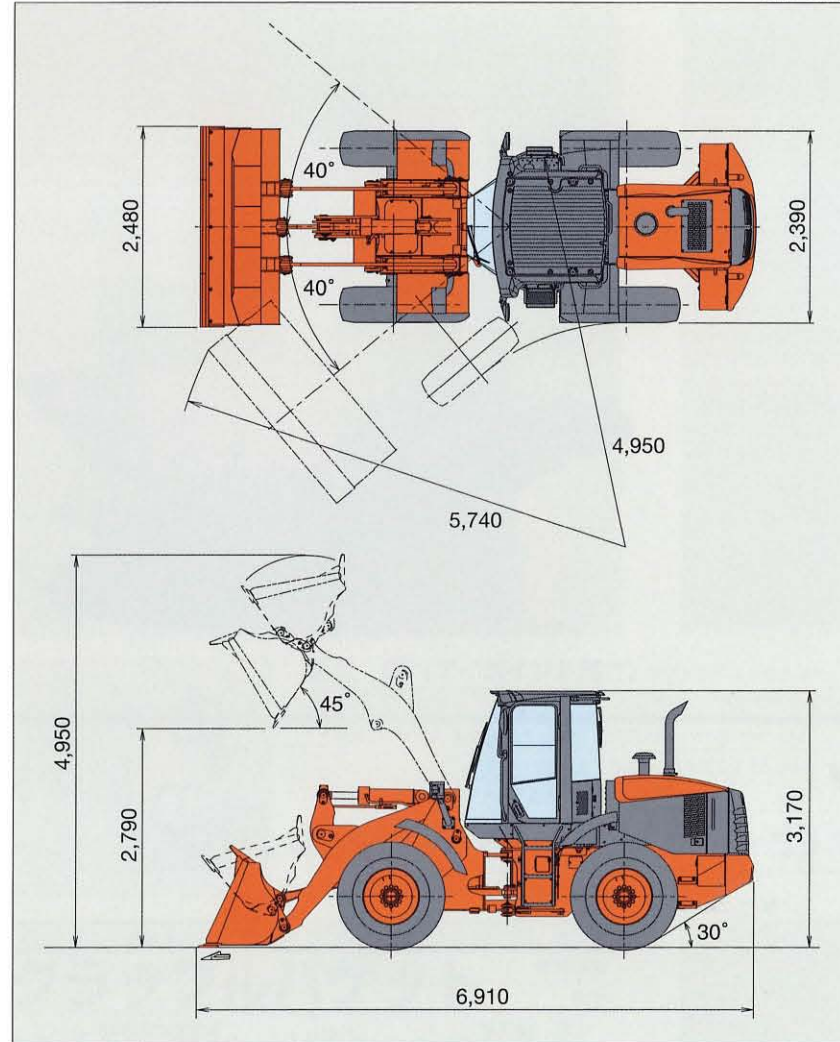
■寸法図 (ZW140)
