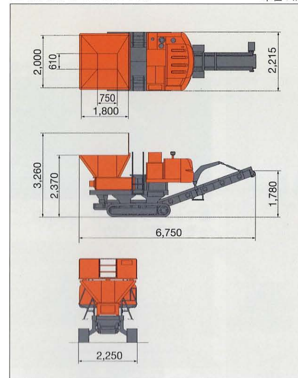
■寸法図 (ZR600TS)
