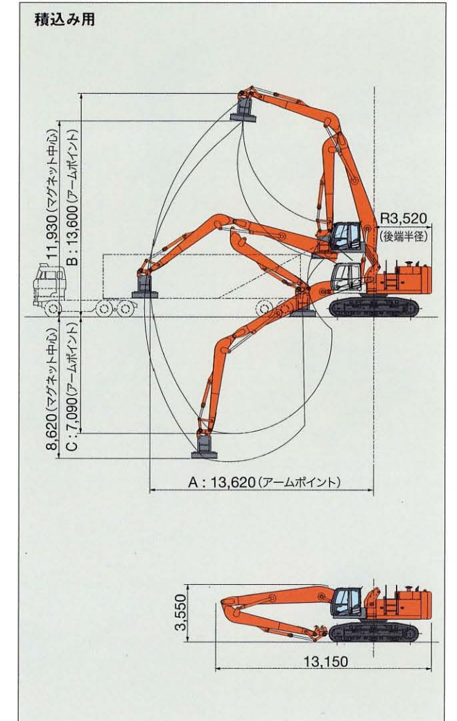
■作業範囲図 (ZX450LC-3)
