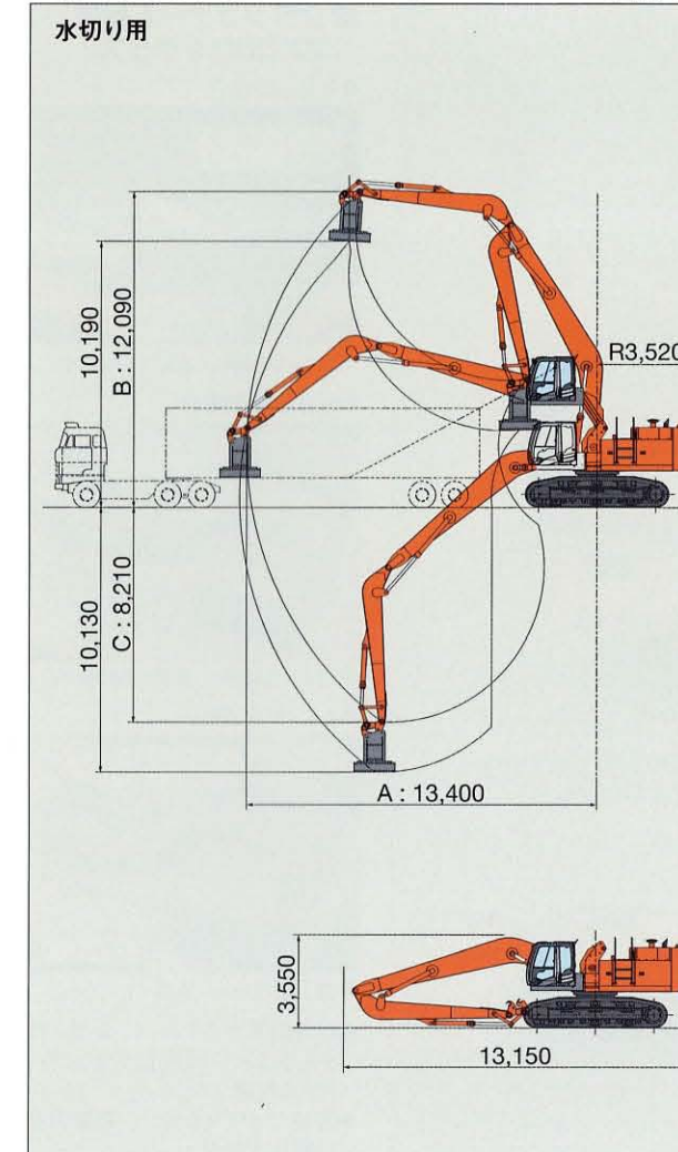
■作業範囲図 (ZX450LC-3)
