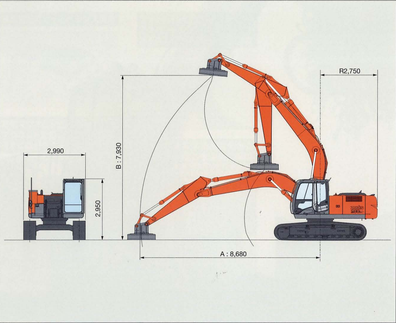
■ 作業範囲図 (ZX200LC-3)
