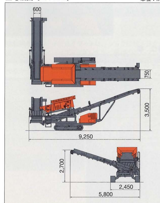
■寸法図 (VR408)
