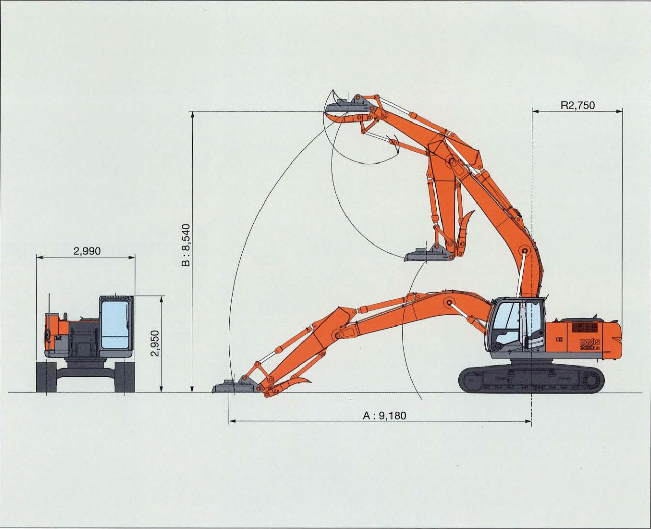
■ 作業範囲図 (ZX200-3)
