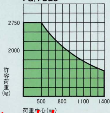
FG/FD28
