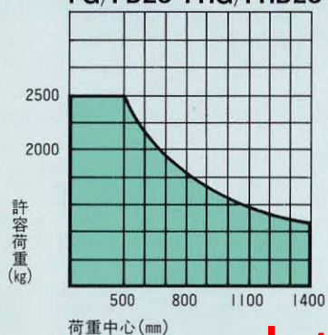
FG/FD25・FHG/FHD25
